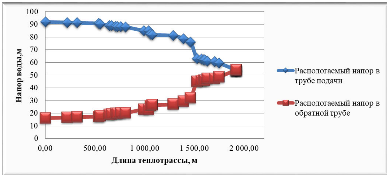
Рисунок 2.5 – Пьезометрический график тепловой сети котельной «Новый Урал» по магистральному выводу
