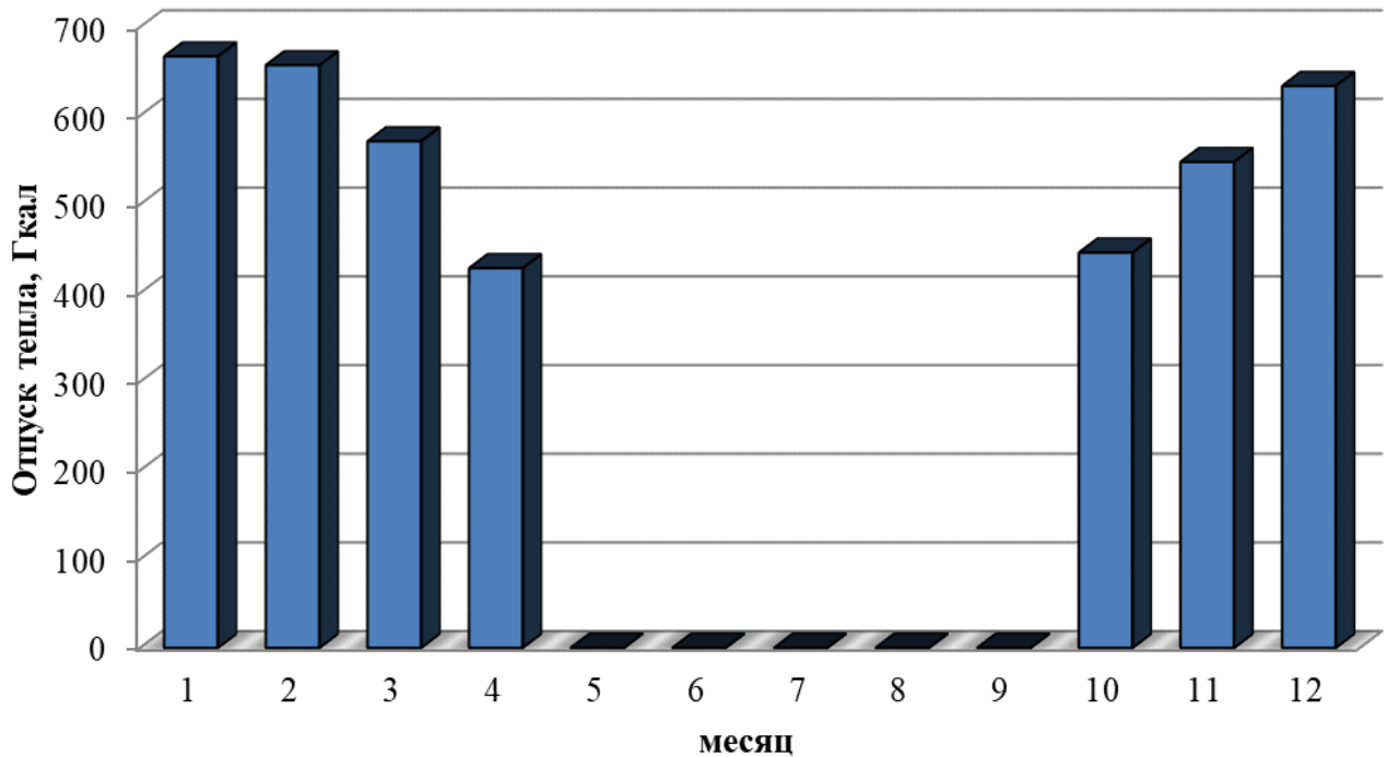
Рисунок 1.2 – Оптимальный температурный график отпуска тепловой энергии для котельной «Новый Урал»
