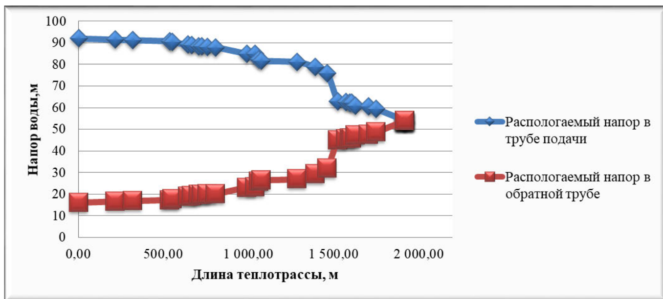
Рисунок 2.4 – Пьезометрический график тепловой сети котельной «Новый Урал» по магистральному выводу
