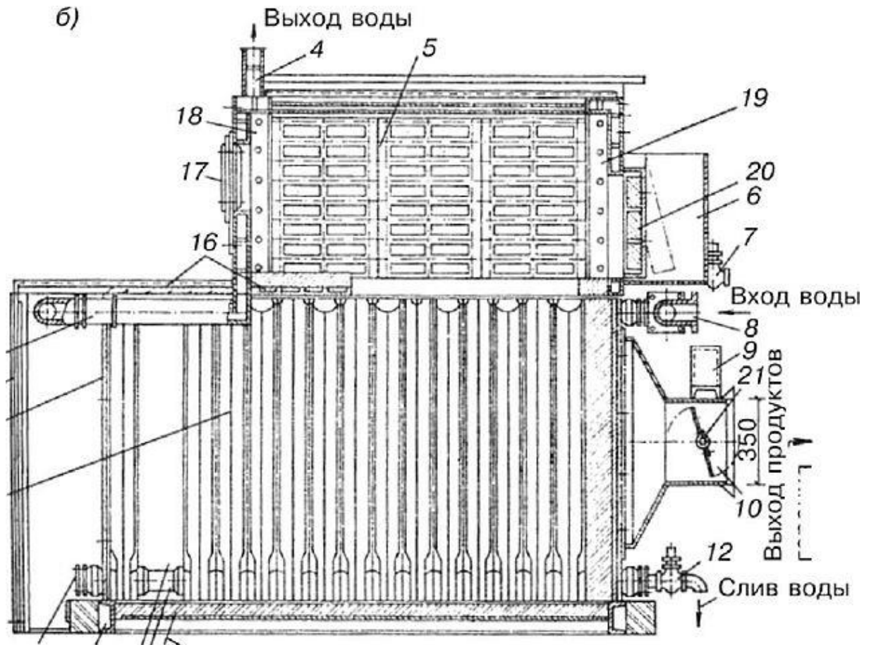
Рисунок 2.1 – Котел Братск-1Г
